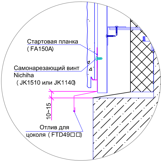
Монтаж оригинального отлива для цоколя Nichiha
