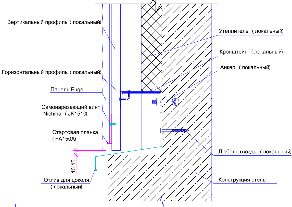
Монтаж оригинального отлива для цоколя Nichiha
